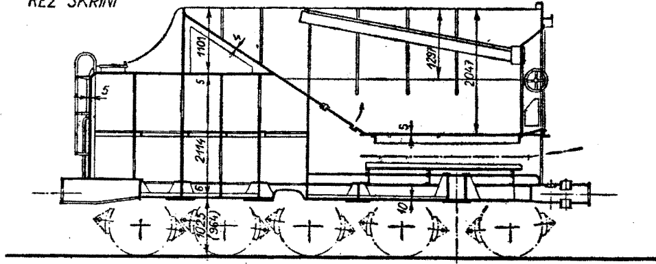
ŘEZ SKŘÍŇI
