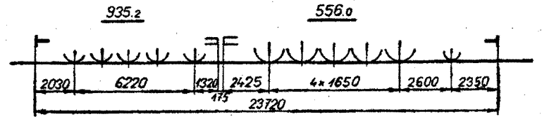
ROZVORY A DÉLKY LOKOMOTIV S TENDRY Ř. 935.2
